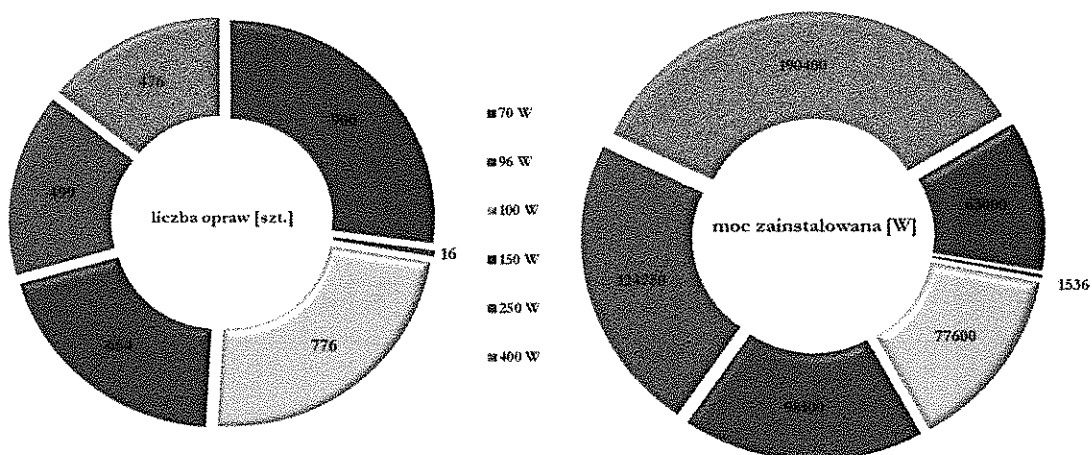
Wykres 22. Liczba opraw oraz moc opraw oświetleniowych
