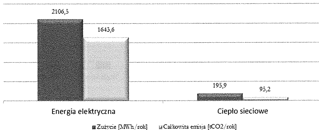
Wykres 31. Wykorzystanie oraz emisja CO 2 z tytułu wykorzystania energii w sektorze komunalnym
