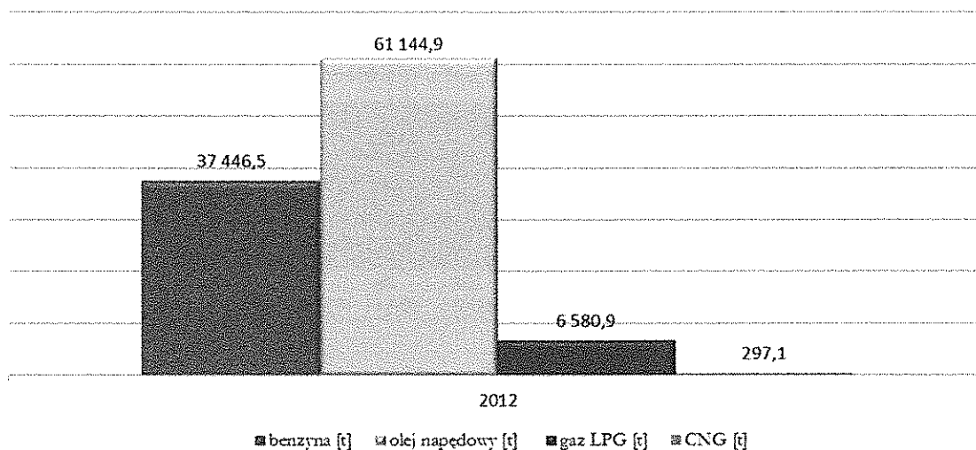
Wykres 42. Bilans energetyczny wykorzystania paliw w sektorze transportu [t CO 2 ]
